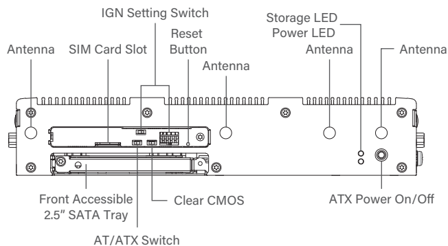
Left I/O
