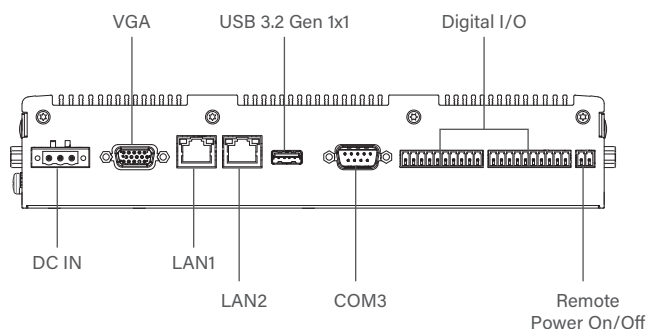
Right I/O
